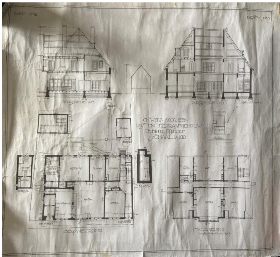
Een kopie van de oorspronkelijke bouwtekeningen met gevelaanzichten, doorsnedes en plattegronden datum 1919
